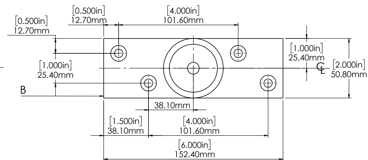
JAMB BRACKET
