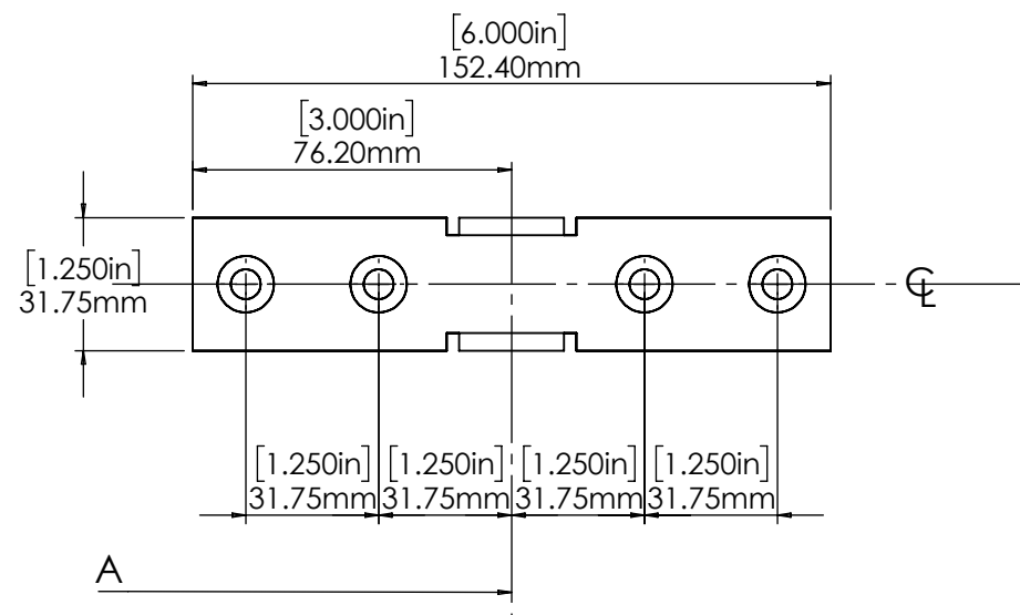
DOOR BRACKET
